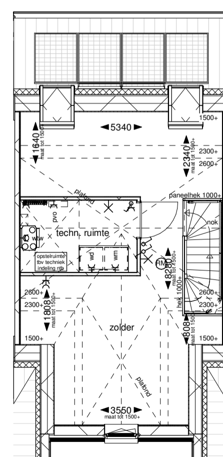
Tweede verdieping
