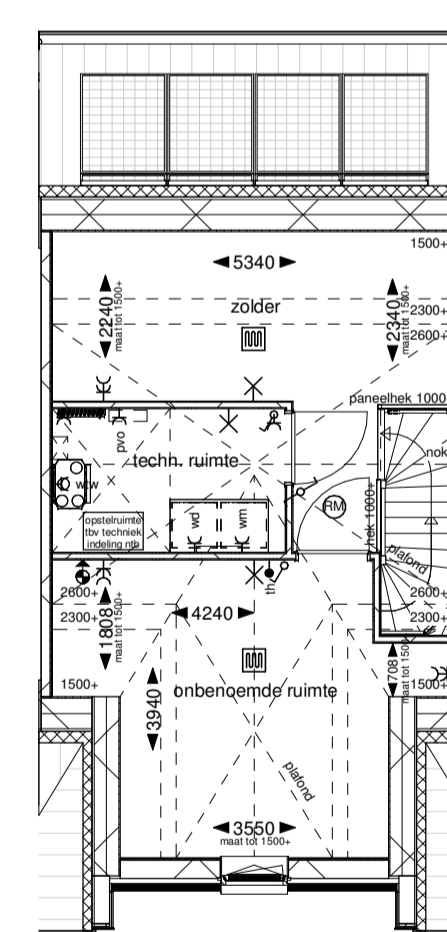
Tweede verdieping
