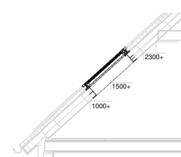
Doorsnede
