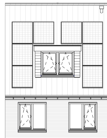
Achtergevel
