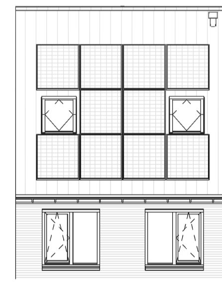
Achtergevel
