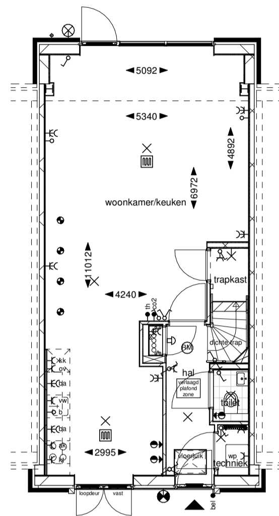
Begane grond
