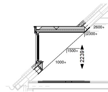
Doorsnede
