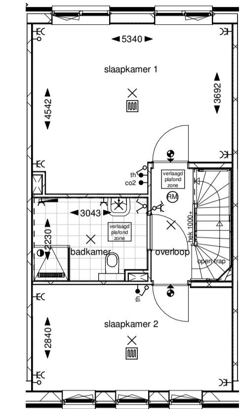
Eerste verdieping
