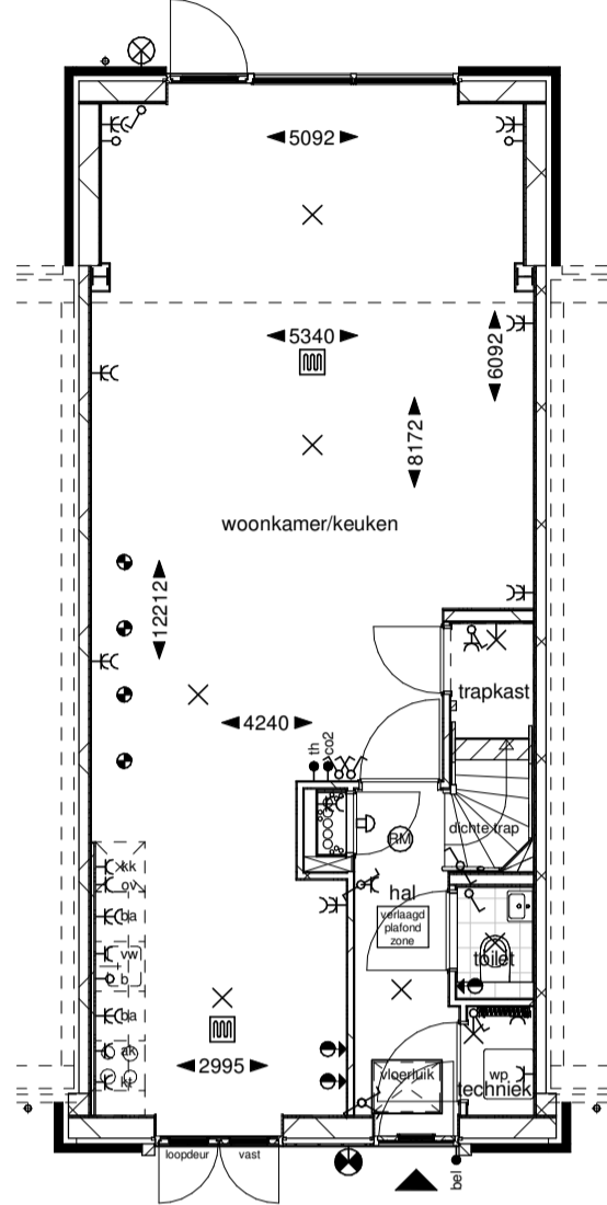
Begane grond
