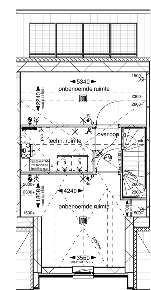
Tweede verdieping
