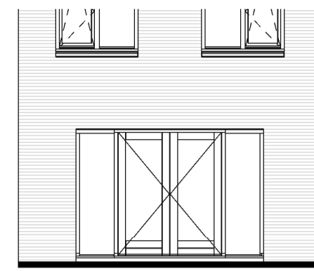
Achtergevel
