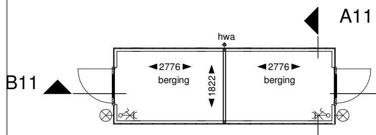
Begane grond
