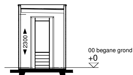
Doorsnede
