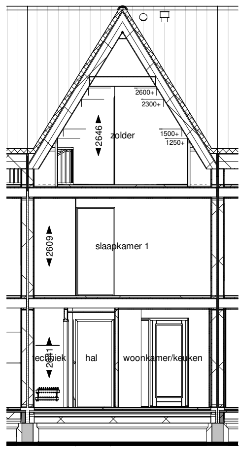
Doorsnede B
