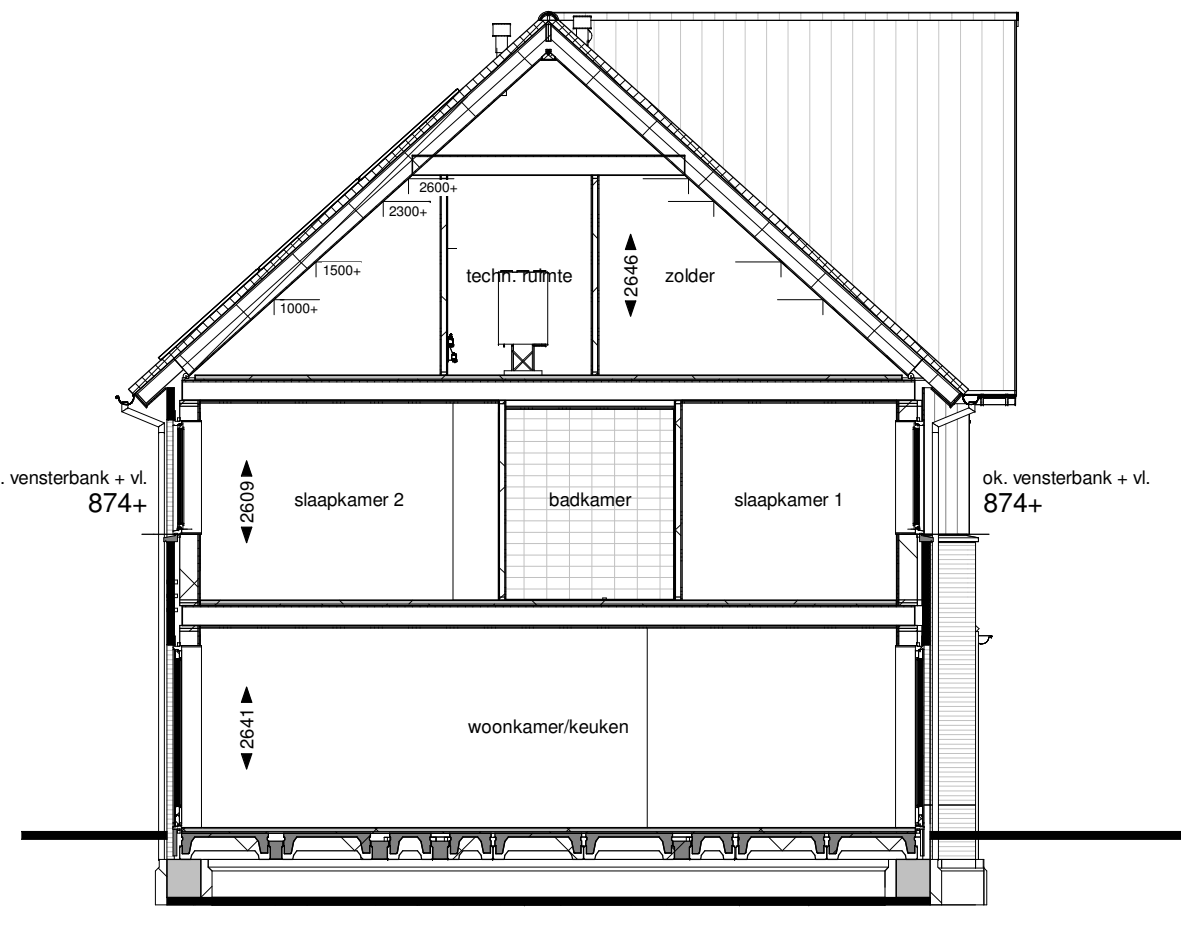
Doorsnede A
